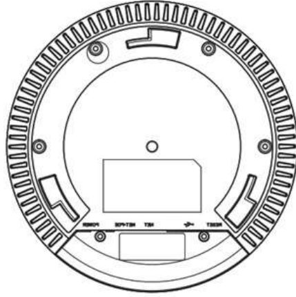
GWN7610/GWN7600 Ports
