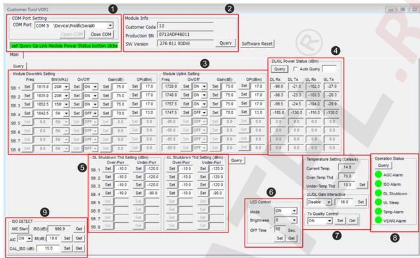
Рис.1 Графический интерфейс пользователя
